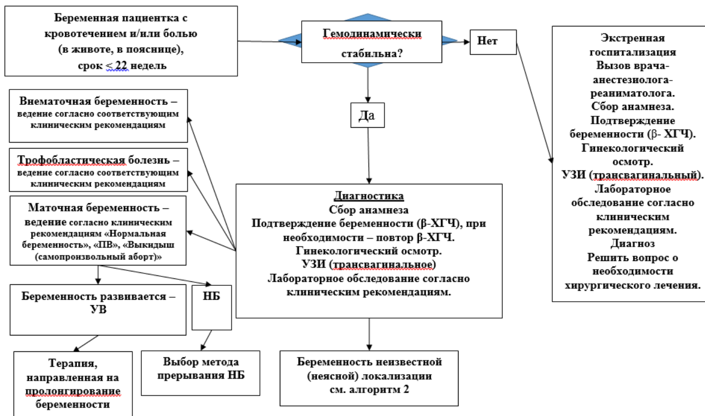
Алгоритм 2. Алгоритм диагностики при беременности неизвестной (неясной) локализации
